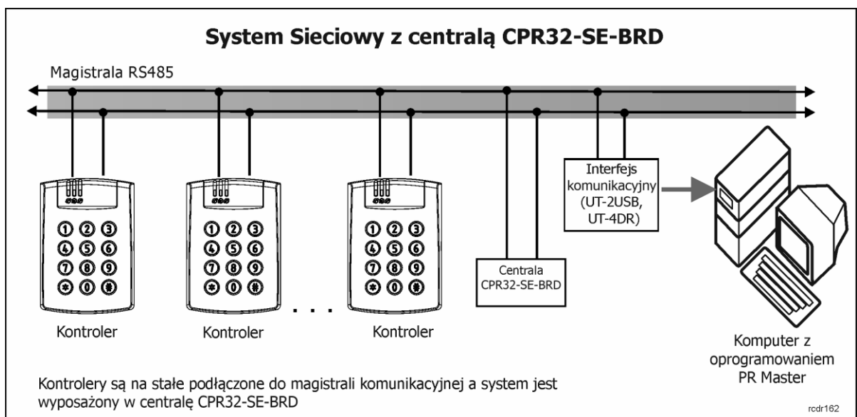
Rys. 4 Praca w Trybie Sieciowym (z centralą CPR32-SE-BRD)
