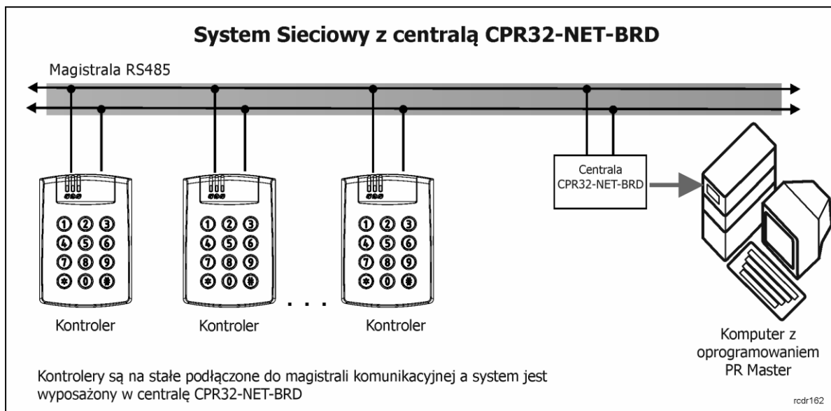
Rys. 5 Praca w Trybie Sieciowym (z centralą CPR32-NET-BRD)
